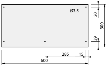
60 × 30 cm fassaadiplaat
