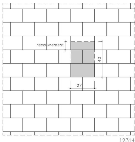
Fig. 1: Format 40/27
