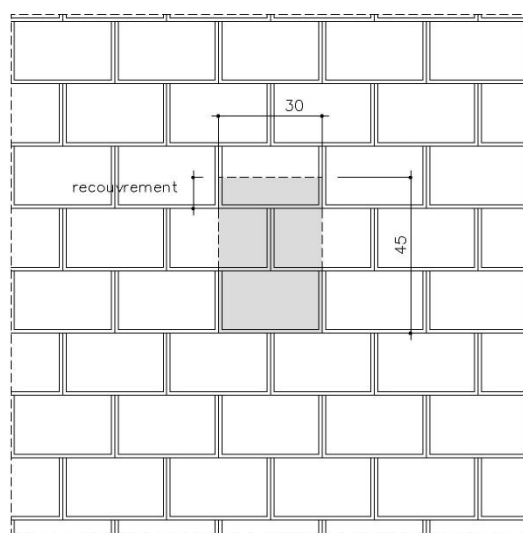
Fig. 8: Format 45/30
