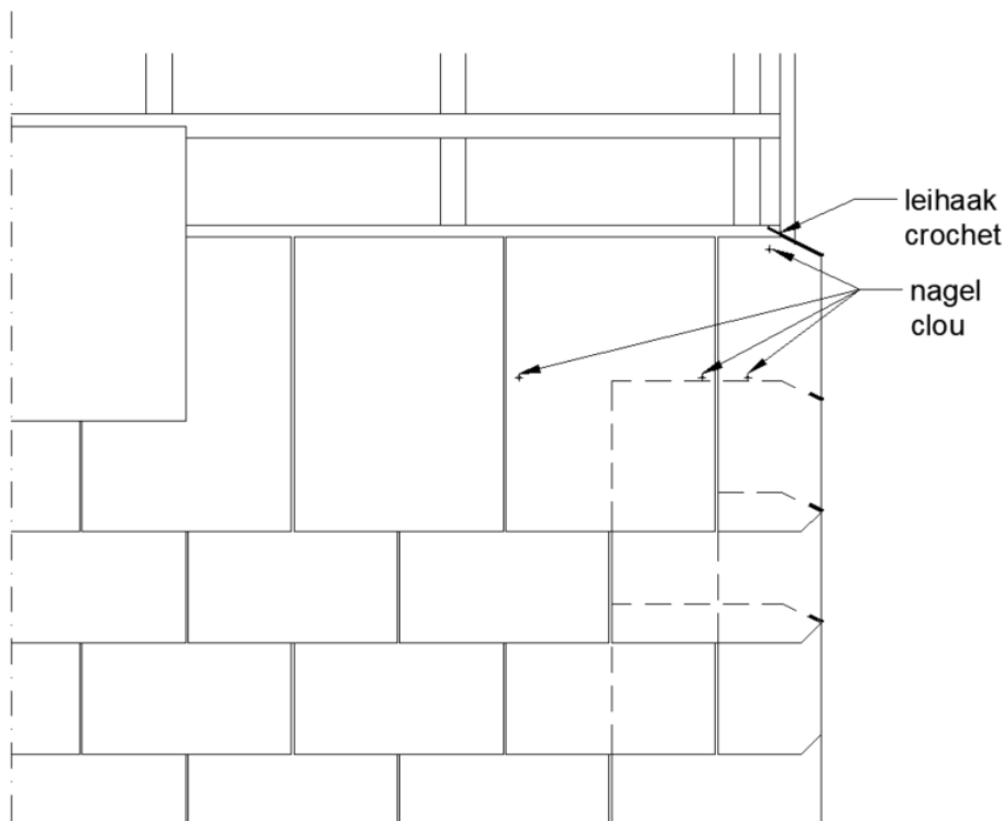
Fig. 19: Rives latérales
