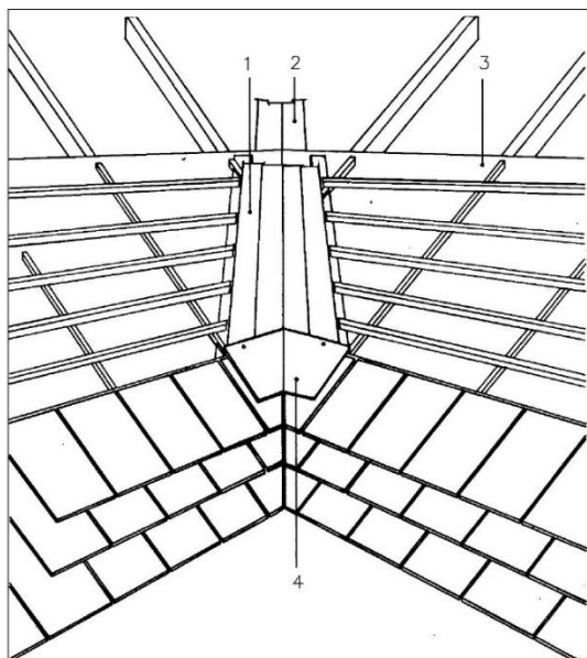
Fig. 17: Noue fermée
